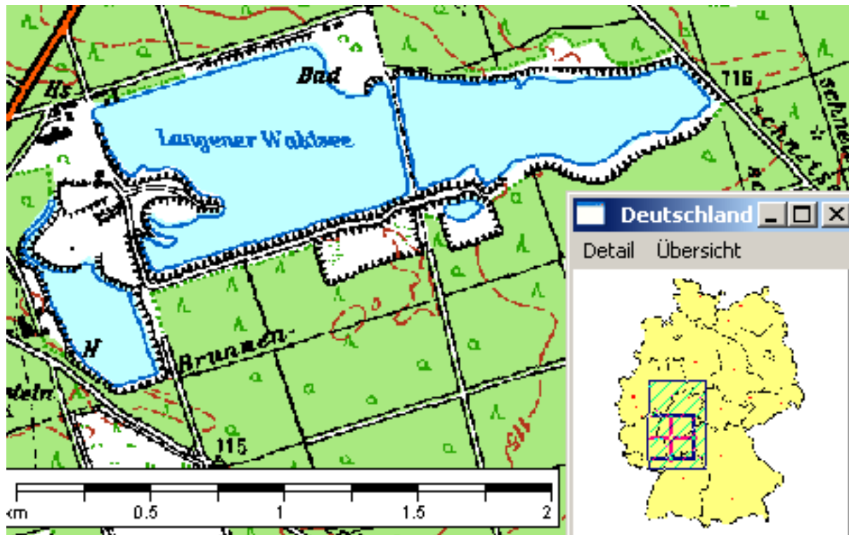
Abb. 1: Ausschnitt aus topographischer Karte (Landesvermessung Hessen 1999)
